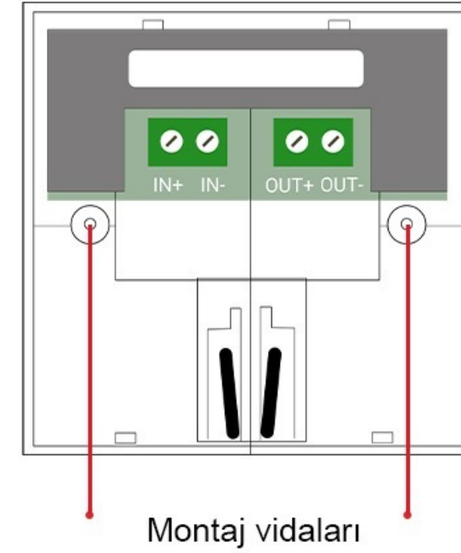
Montaj vidaları
